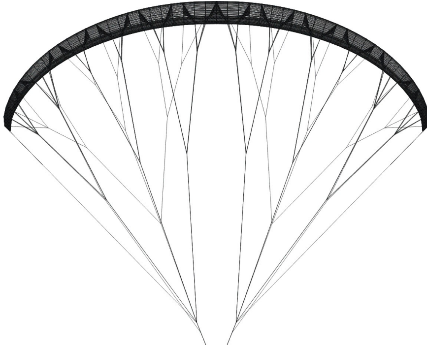
Bild 1: Gittermodell Mistral 5 (Frontansicht)
