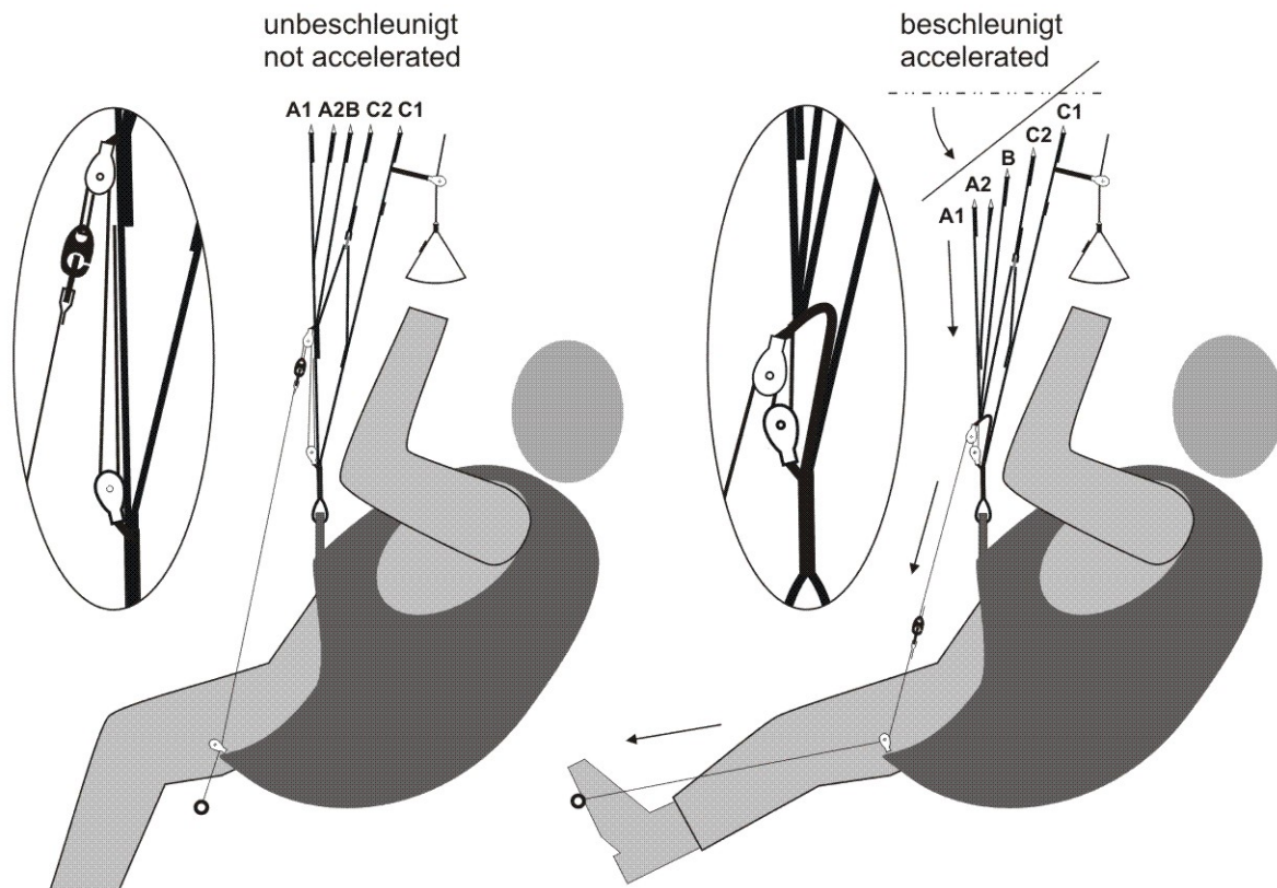
Bild 2: Funktionsweise Fußbeschleuniger Mistral 5
