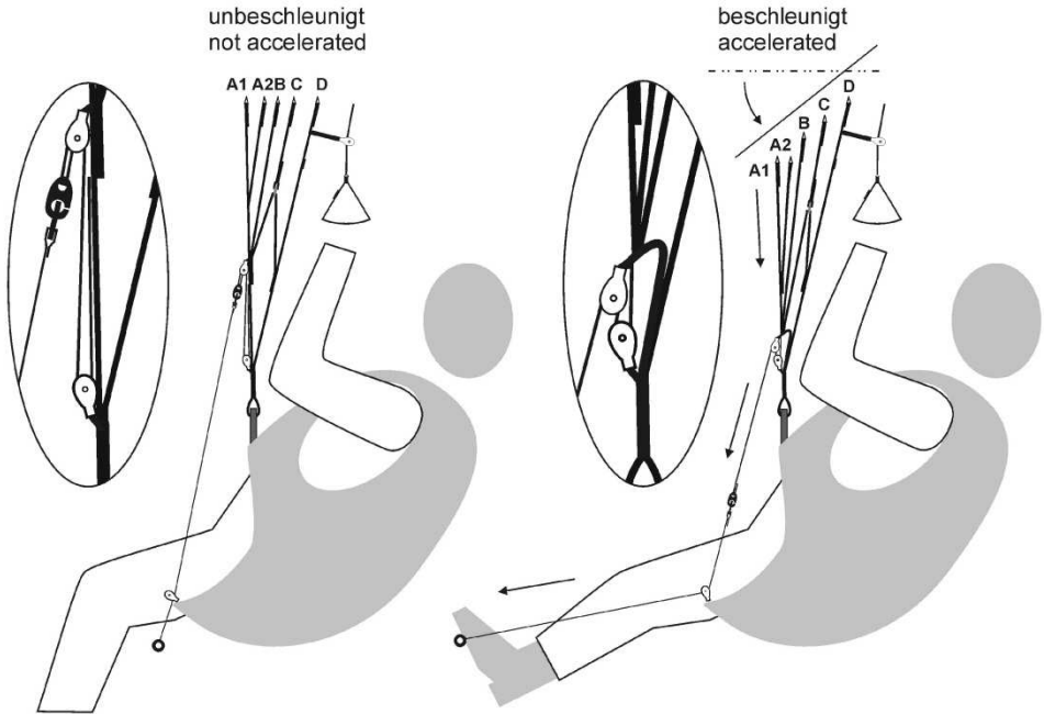
Abbildung 5: Funktionsweise Fußbeschleuniger Arcus 7
